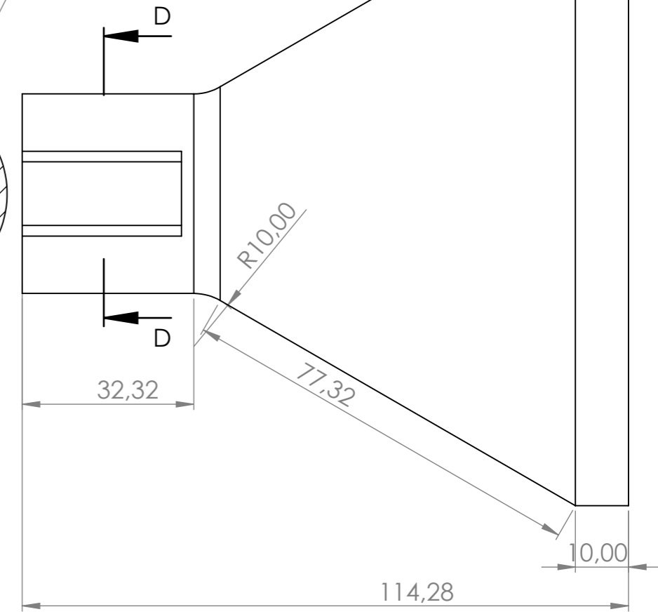
SECTION D-D SCALE 1 : 1
